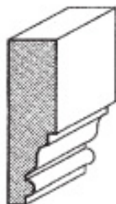
EC12 APRON 1 1/16" x 2 1/2"
